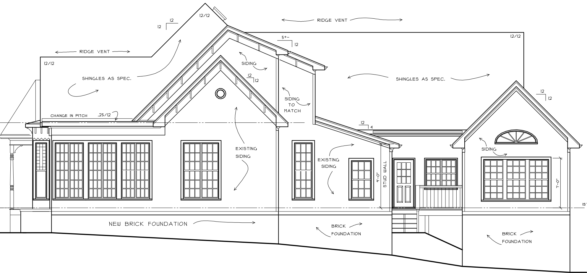
RIGHT ELEVATION
